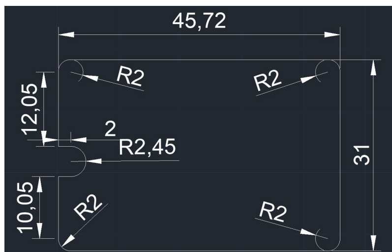
PCB 尺寸图 (长 45.72mm,宽:31mm,高 1mm)
